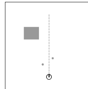
Map m
