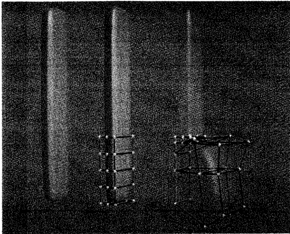
Fig. 14 Local FFD
